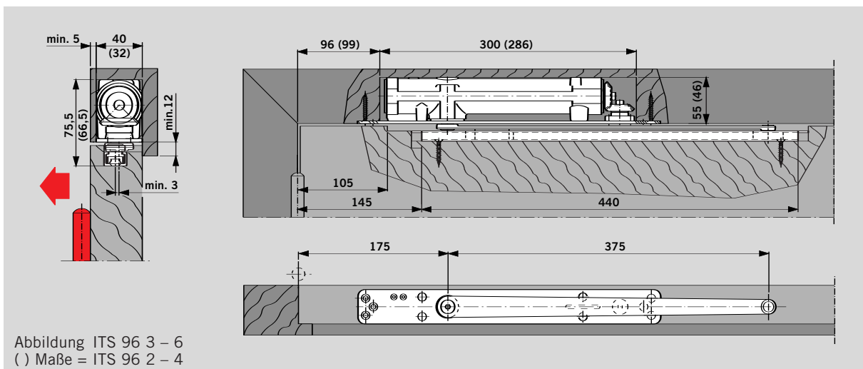
Türschließer DORMA ITS 96 mit Gleitschiene DORMA G 96 N20 in einer Holz Kopfmontage Beispiel: DIN-L-Tür, DIN-R-Tür spiegelbildlich
