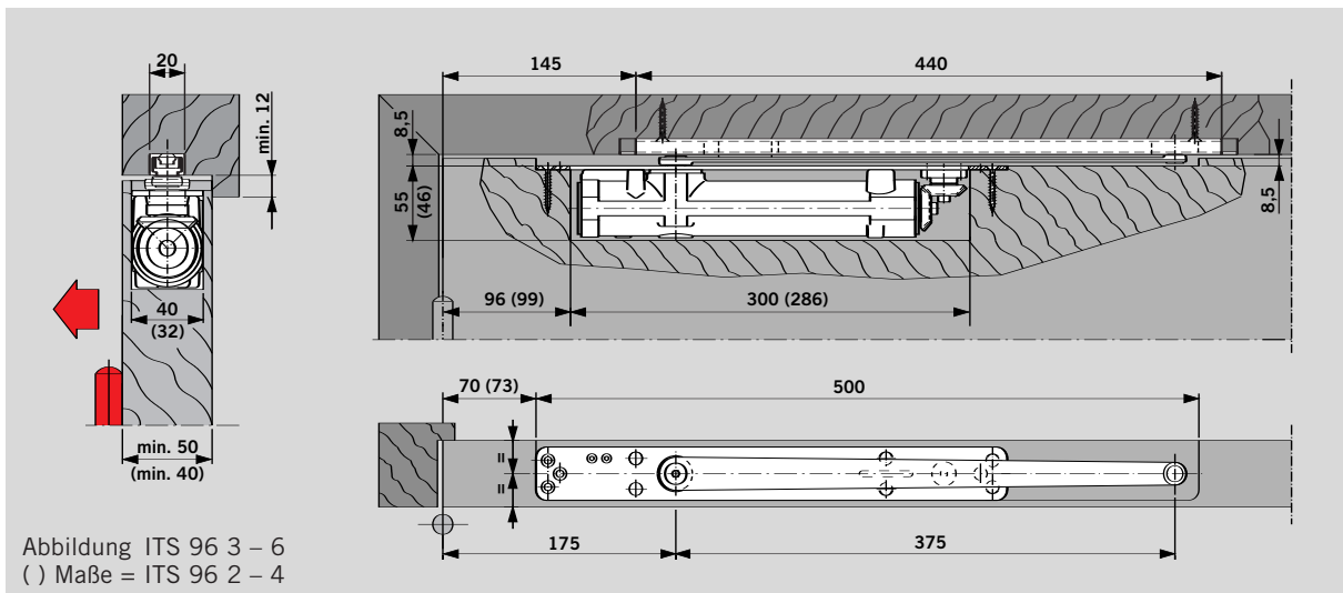
Türschließer DORMA ITS 96 mit Gleitschiene DORMA G 96 N20 in einer Holz tür Beispiel: DIN-L-Tür, DIN-R-Tür spiegelbildlich
